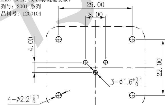
线路板开板尺寸 (未注公差 \pm 0.1 ) 俯视图
