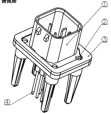
3D 视图
