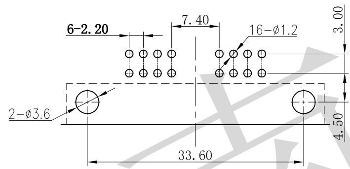
线路板开板尺寸 (未注公差±0.1) 俯视图
